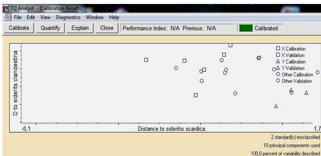
Εικόνα 4.7 Διαχωρισμός των φύλλων/βρακτίων εξομαλυνθέντων φασμάτων απορρόφησης με βάση τη βοτανική ταξινόμηση του Sideritis στις περιοχές 1.484-1.297 \text{cm}^{-1} και 1.195-935 (δεύτερη παράγωγος)
