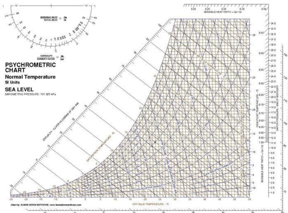
Σχήμα 41: Ψυχομετρικό διάγραμμα σε μονάδες SI
